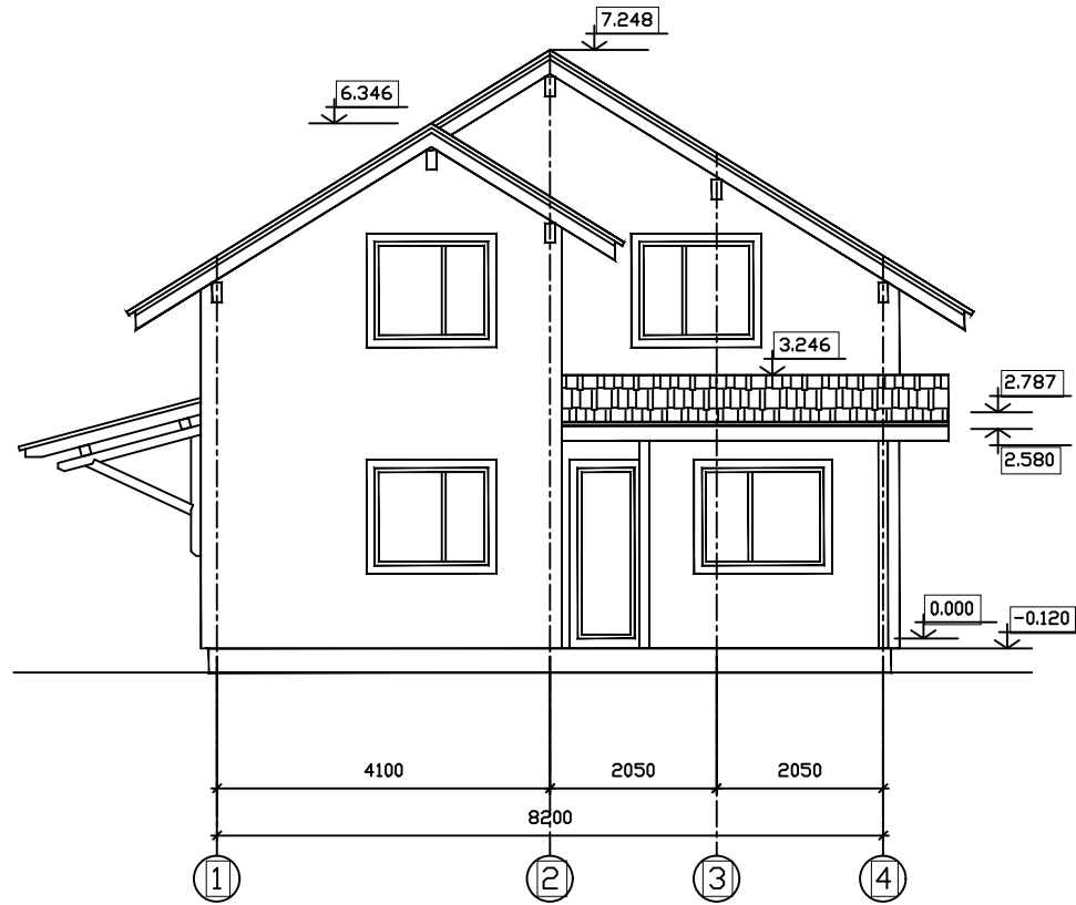
Фасад 1-4
